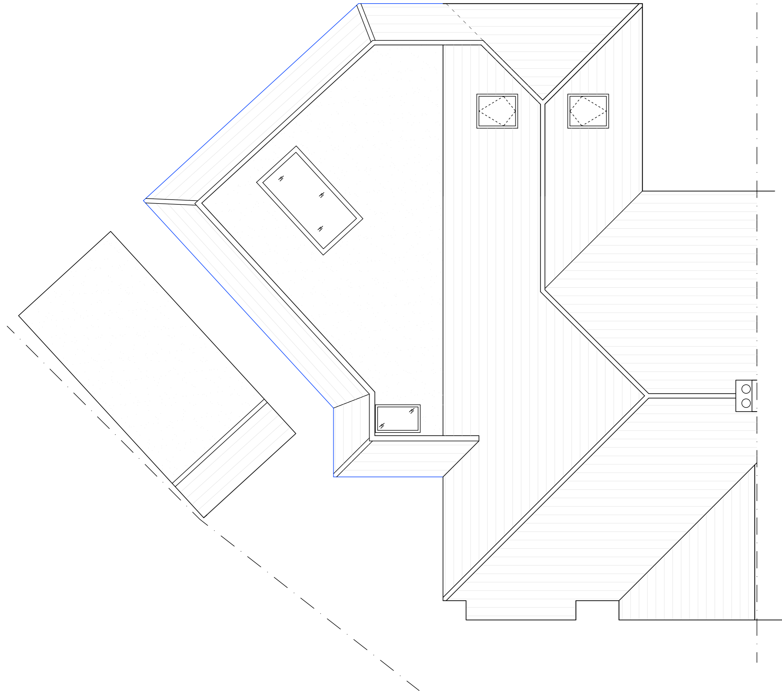
○ Roof Plan 1:50
