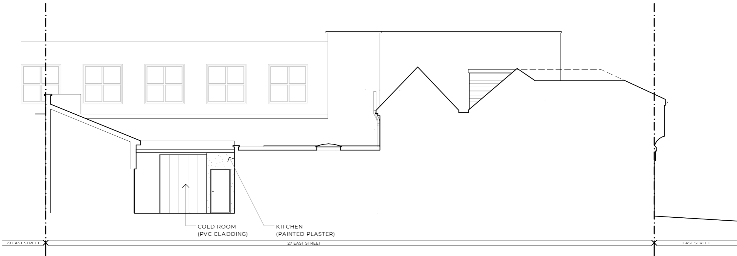
1 Existing - Elevation E2
