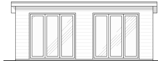
04 south elevation Scale: 1:100
