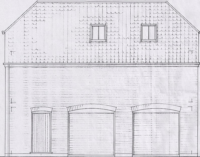
FRONT ELEVATION (N.W.)
