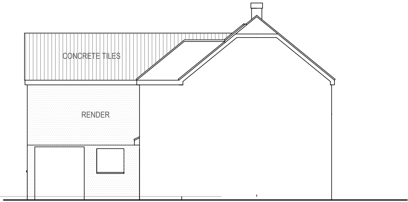
RHS ELEVATION
