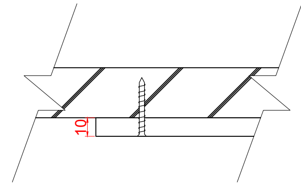
DETAIL 'A' 1:2
