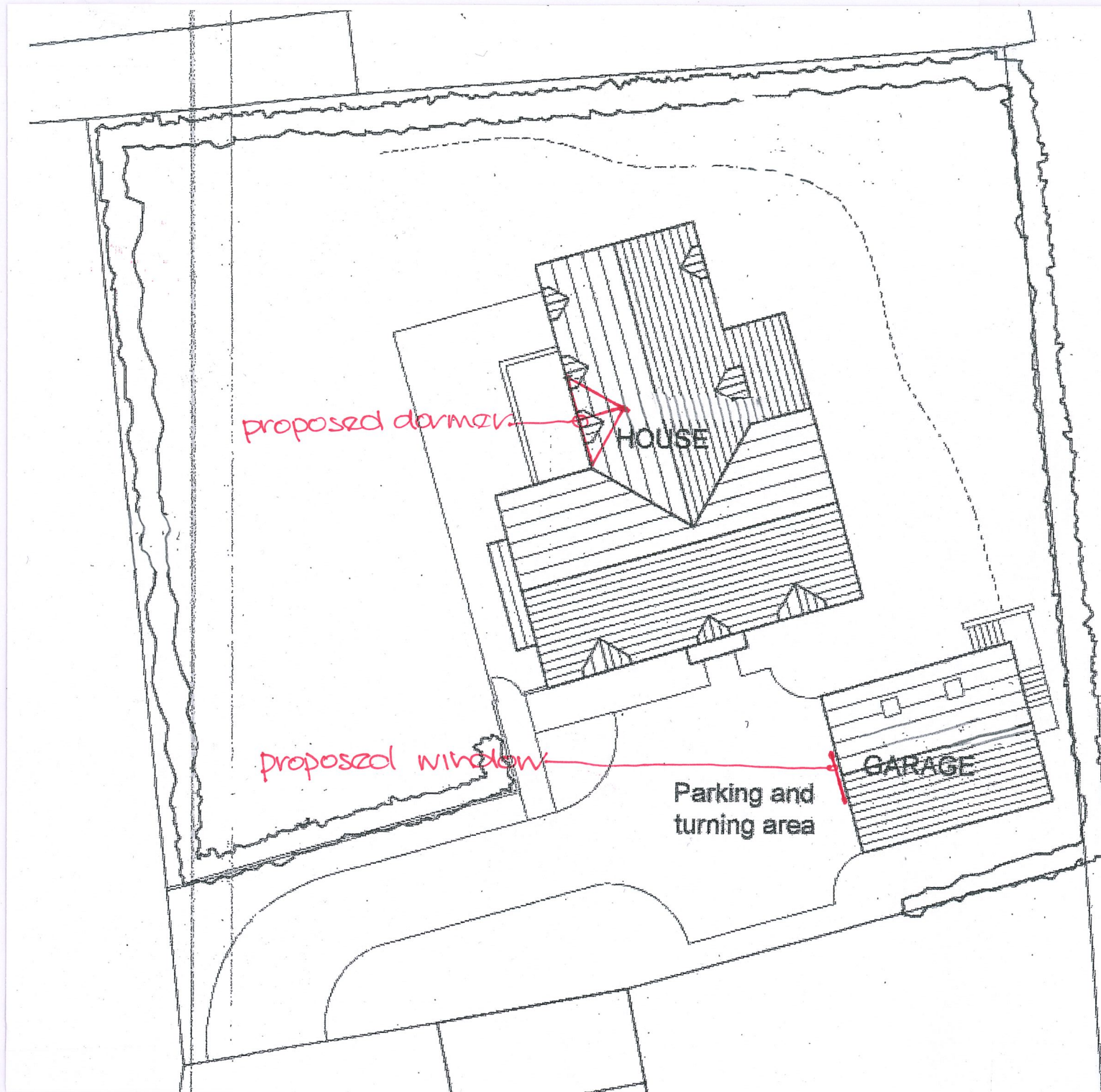
SITE PLAN 1:200.
