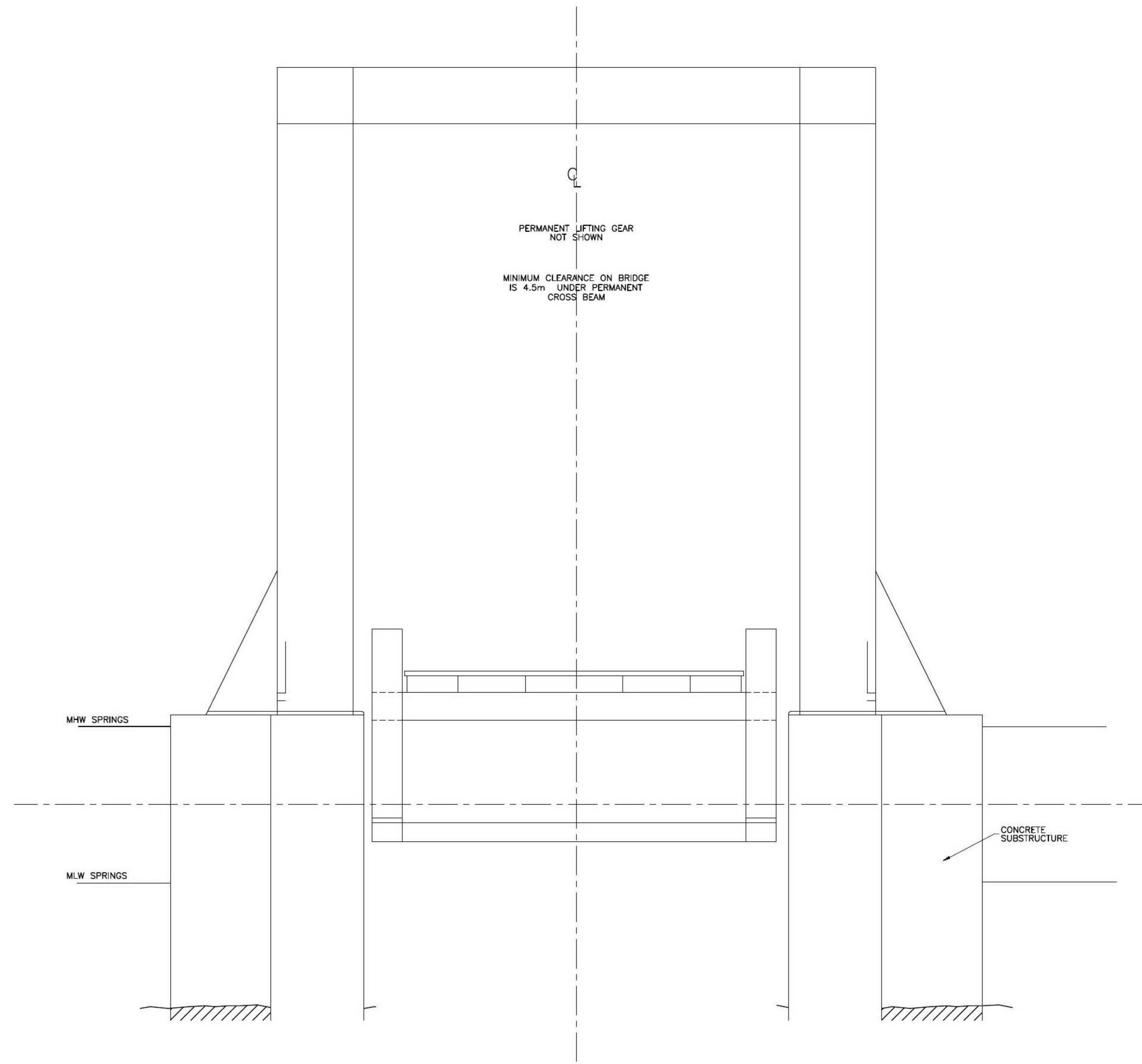
SECTION A-A
