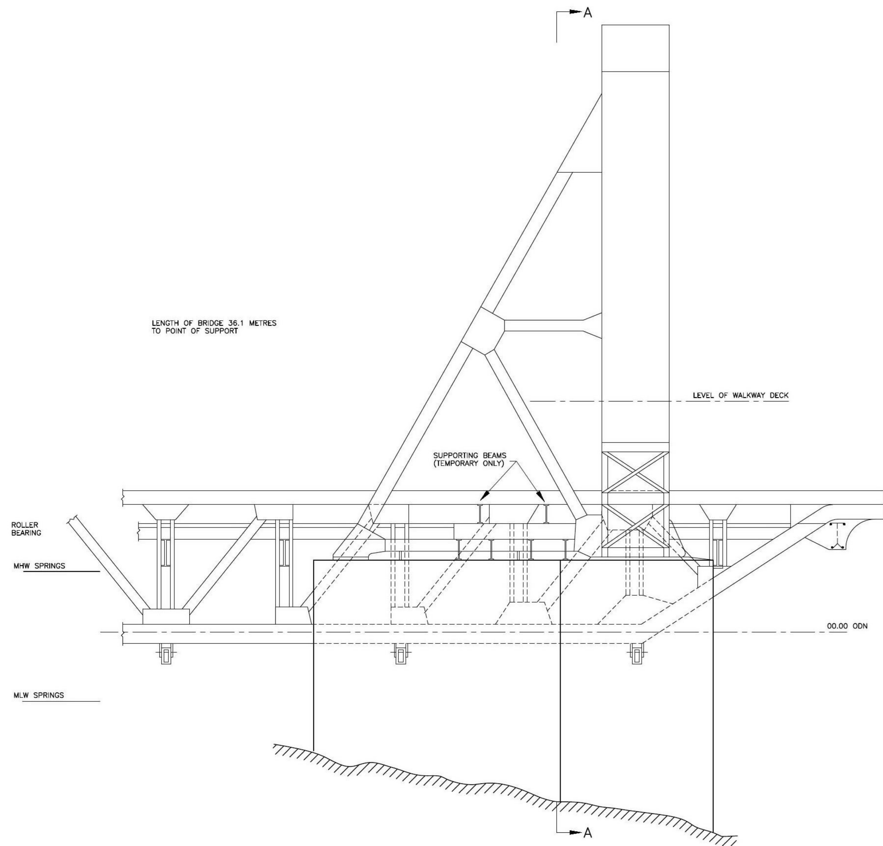
ELEVATION
