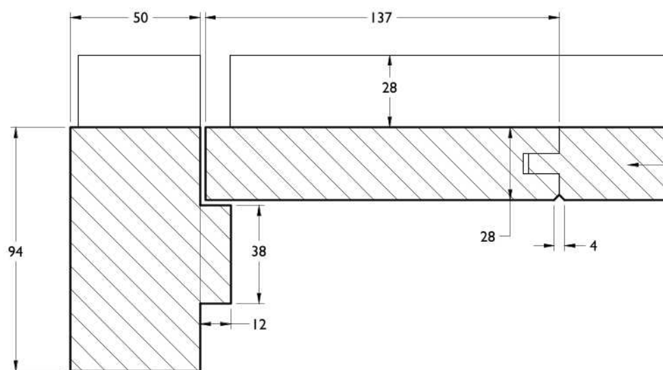
PLAN AT A. JAMB DETAIL. 1:2
