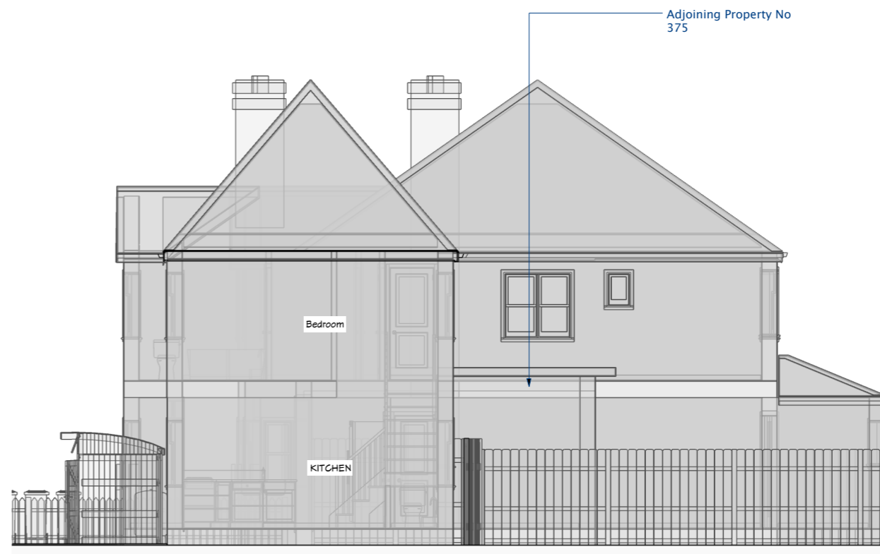
Right Elevation
