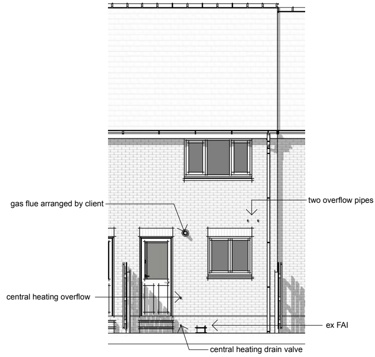
E :: EXISTING REAR ELEVATION 1 scale: 1:100
