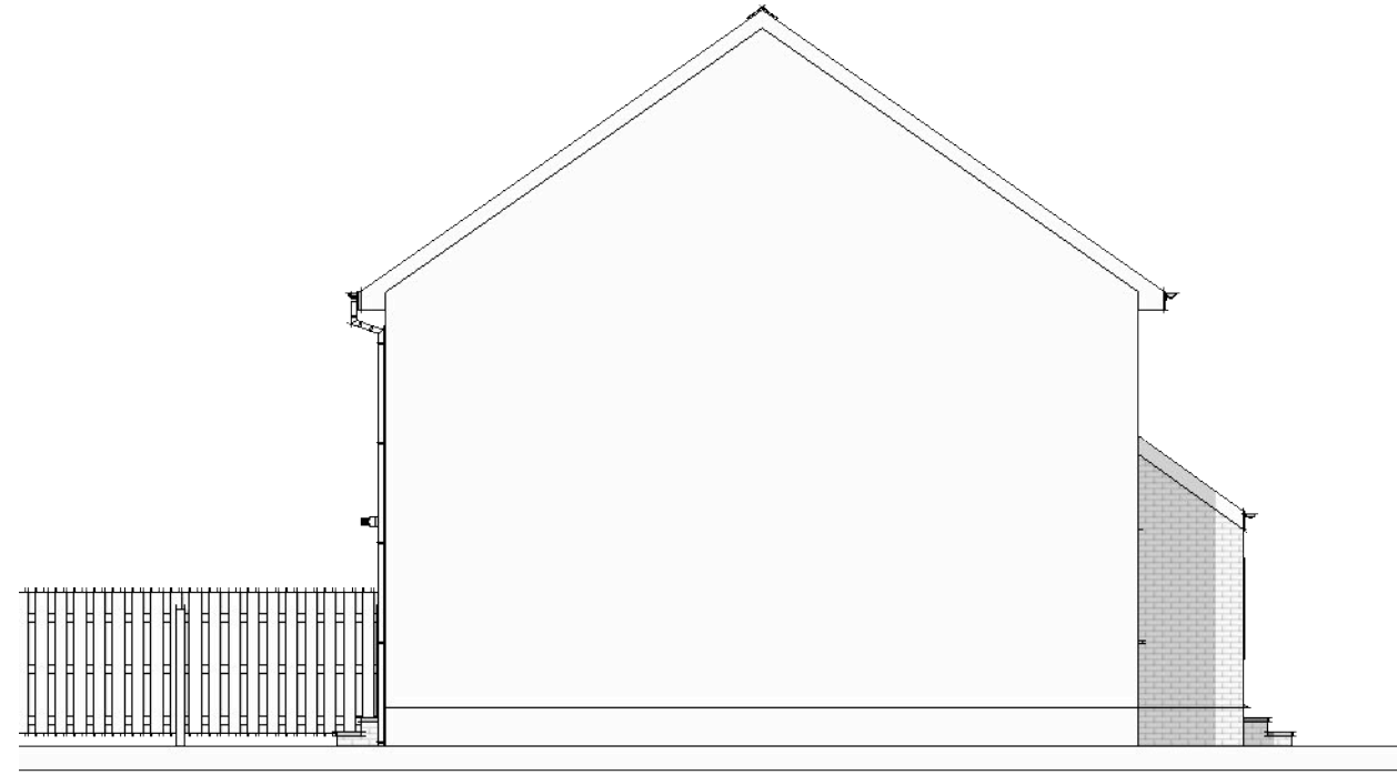
E :: EXISTING SIDE ELEVATION 1 scale: 1:100
