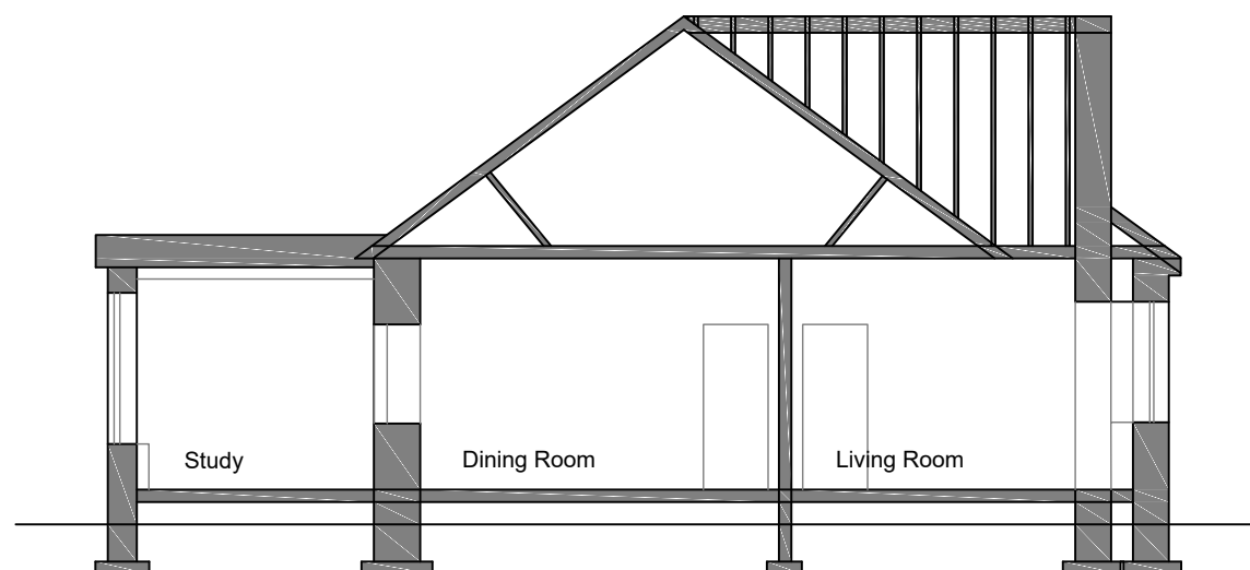
Section BB 1 : 100
