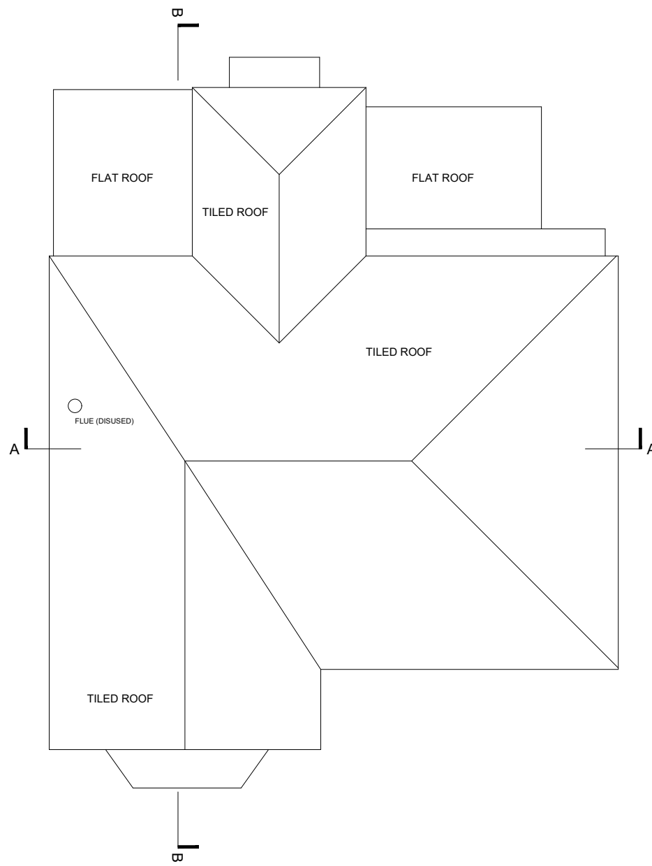
Roof Plan 1 : 100
