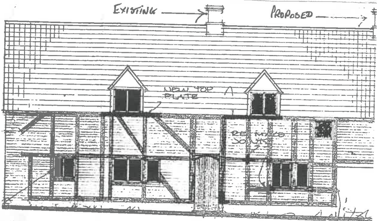
S.E. ELEVATION
