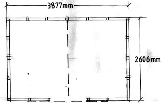
PLAN 1:50
