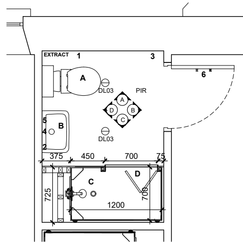
STAFF ENSUITE PLAN
