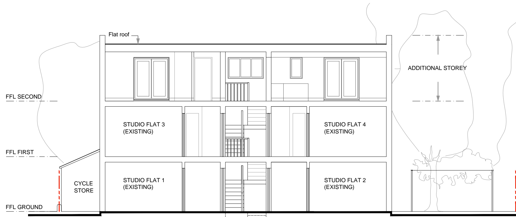
SECTION A-A
