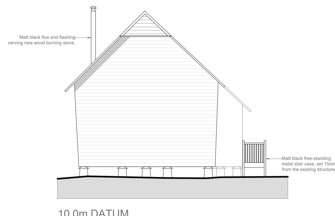
10.0m DATUM EAST ELEVATION BARN B
