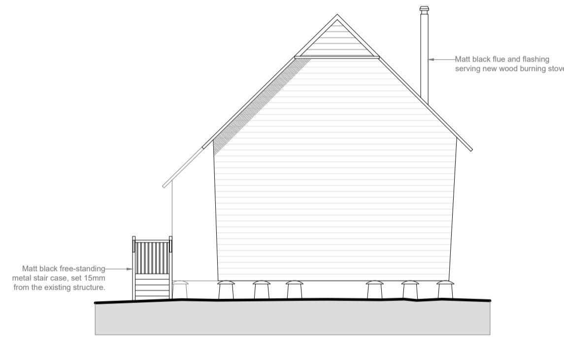
10.0m DATUM WEST ELEVATION BARN B
