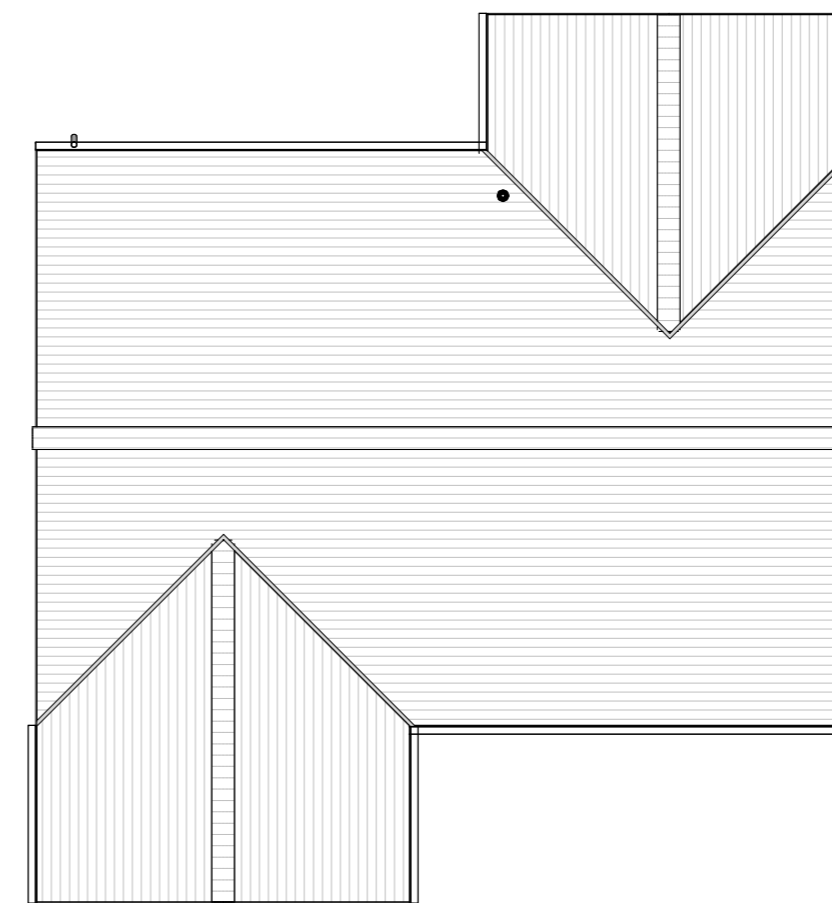
Roof Plan 1 : 100
