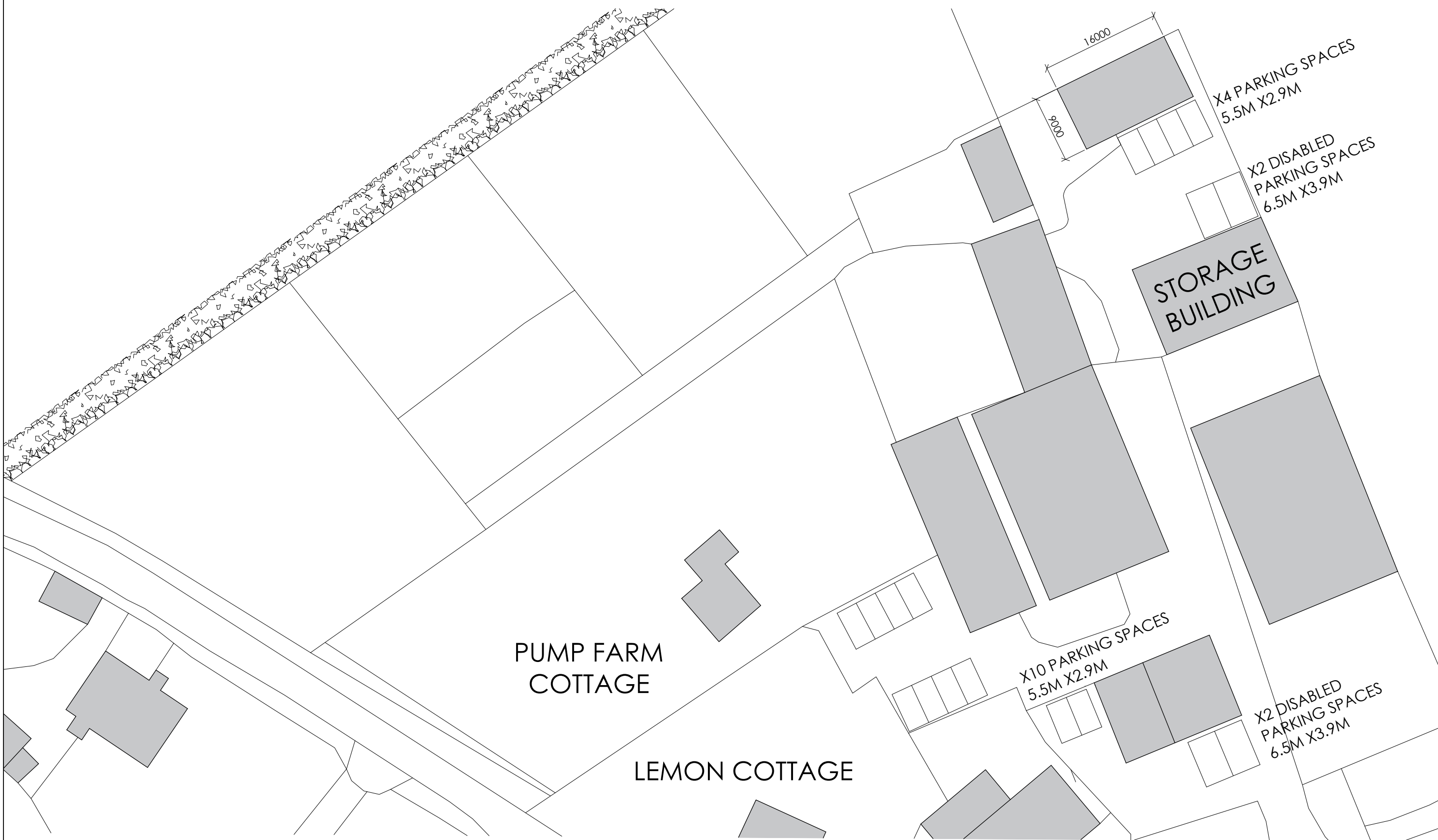
1 SITE PLAN SCALE: 1:500 @ A3
