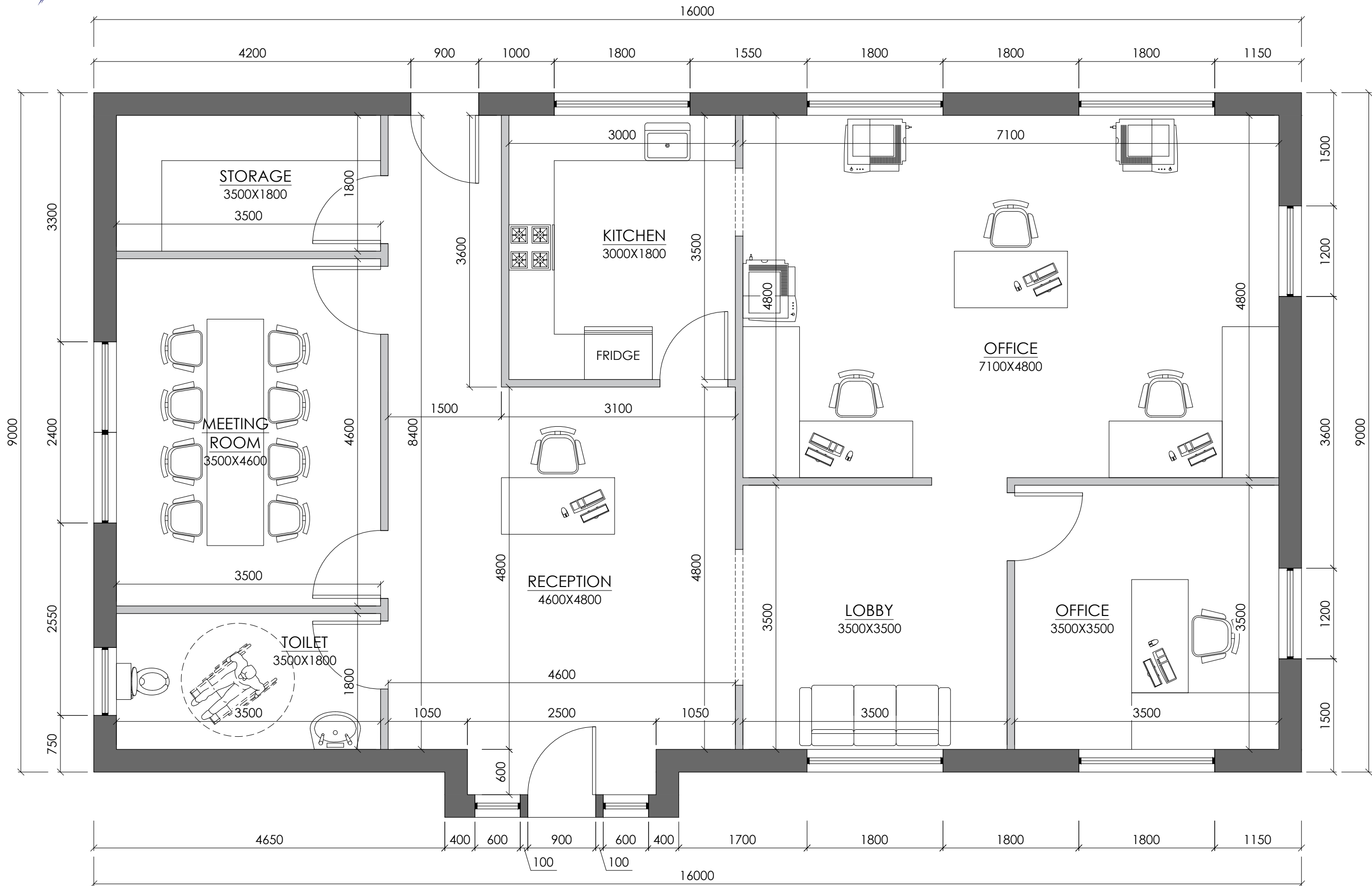
1 FLOOR PLAN SCALE: 1:50 @ A3
