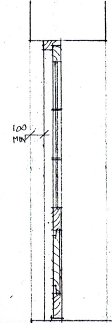
SECTION D4
