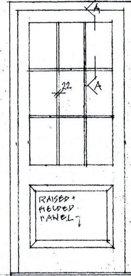
D4 SCALE 1:20
