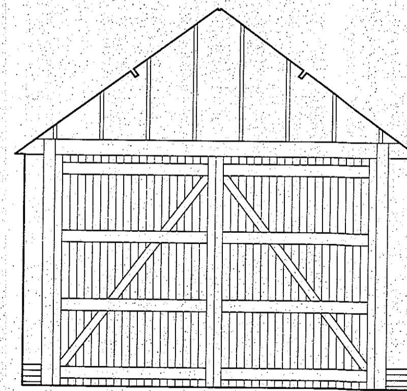
ELEVATION 4
