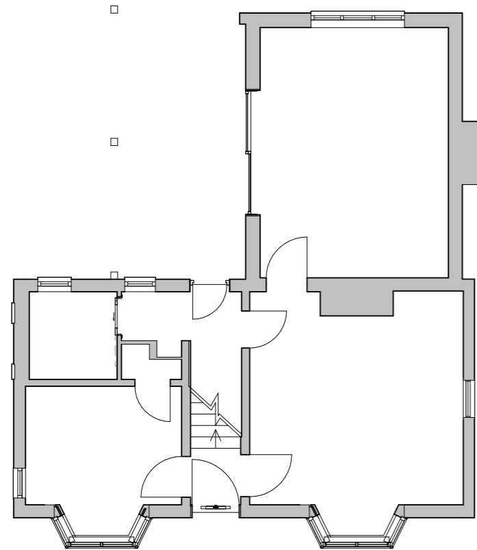
Existing - GF 1 : 100
