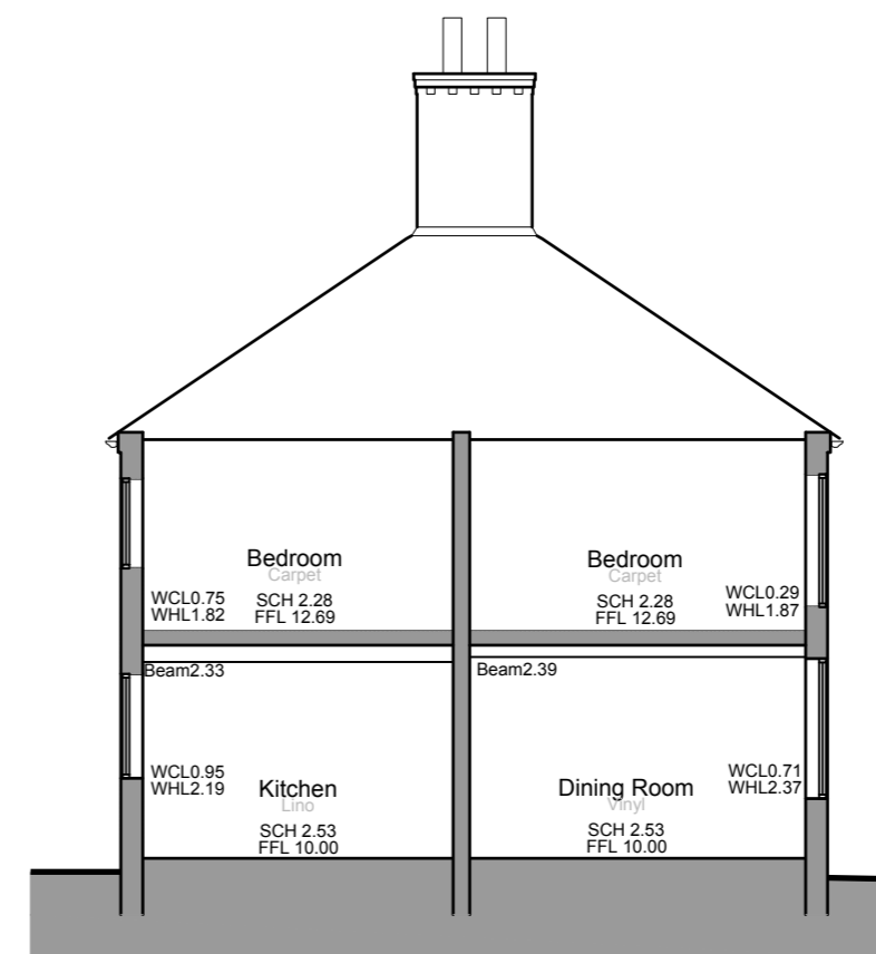
Section B-B 1:100 - A1
