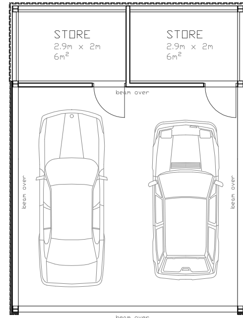
CARPORT 1 (PLOTS 1+2)
