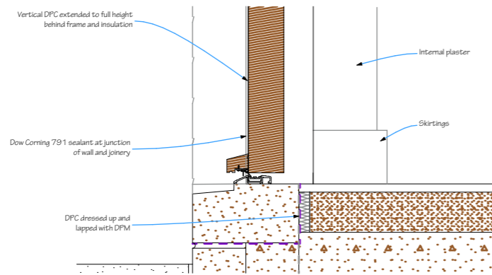
4 DOOR SECTION 1:10
