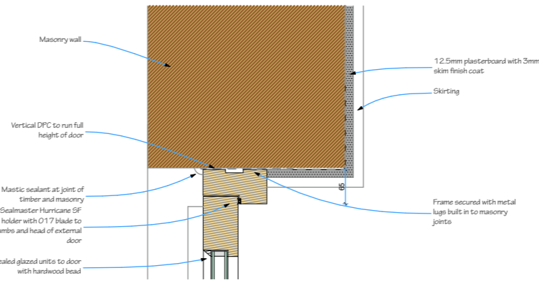
3 DOOR JAMB 1:10
