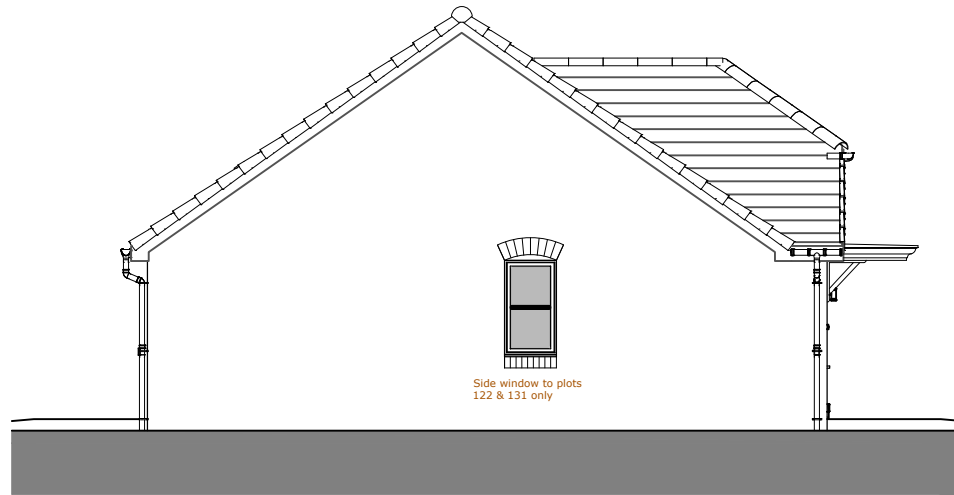
L.H. SIDE
