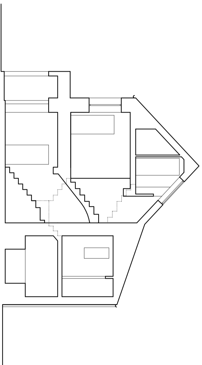
1 Section A-A
