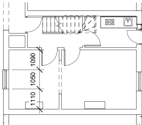
1 Level 0 0 1 : 100
