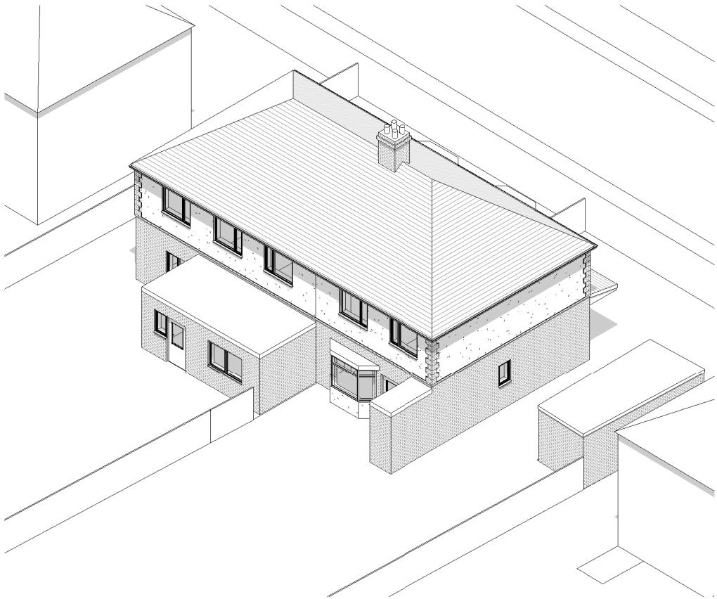
P-004 - EXISTING AXO
