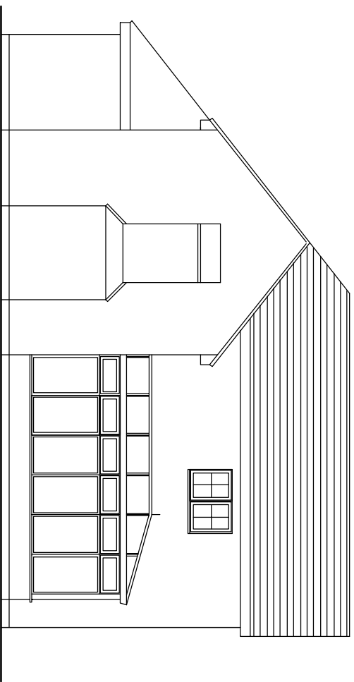
EXISTING FLANK ELEVATION
