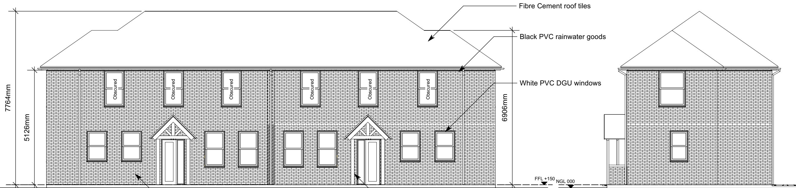
1 East Elevation Scale: 1:100
