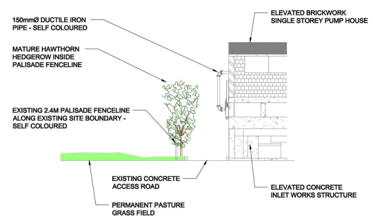
SECTION B 1:100 Y01-102
