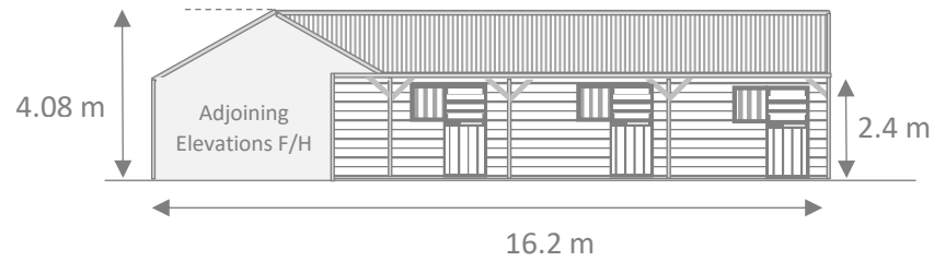
ELEVATION I
