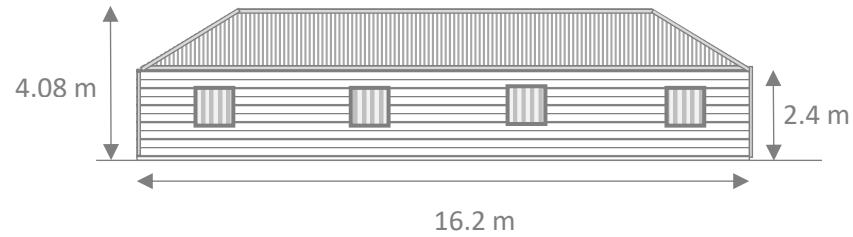
ELEVATION J
