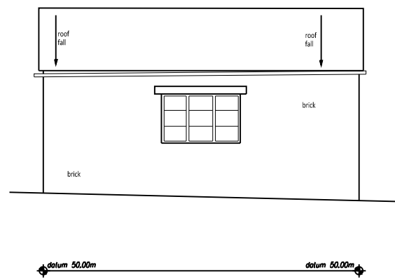
Elevation E9
