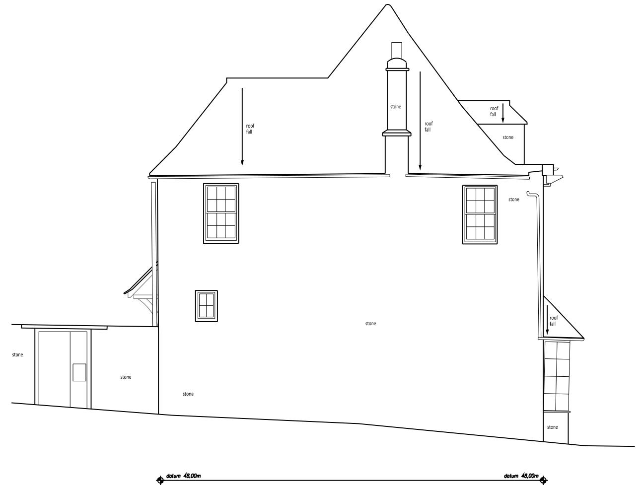
Elevation E2
