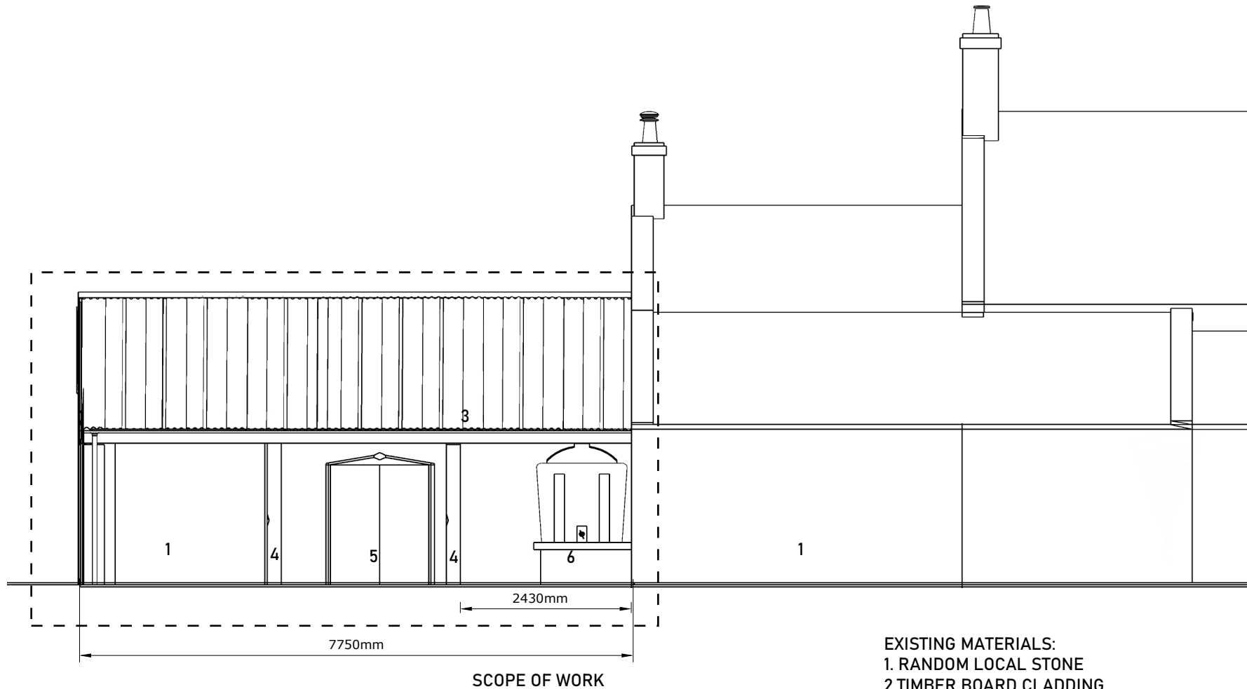
ORTH ELEVATION
