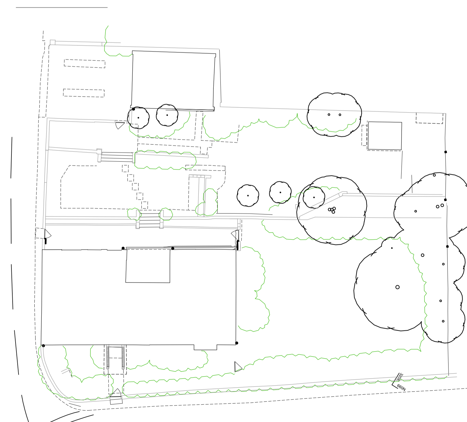
6 Site Plan 1 : 200
