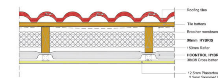
U-value 0.18 W/m 2 K
