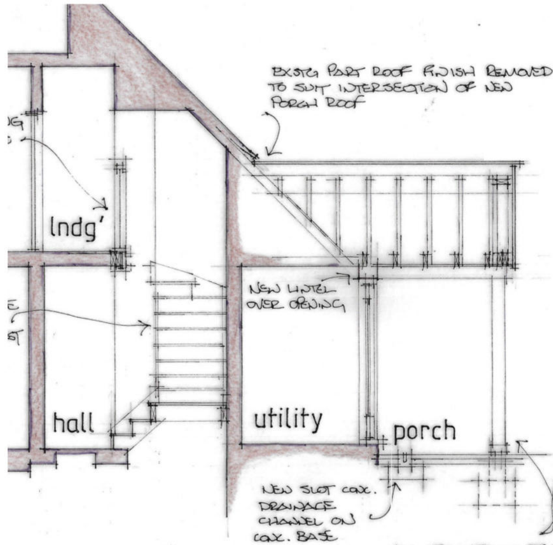
Section A-A 1:50
