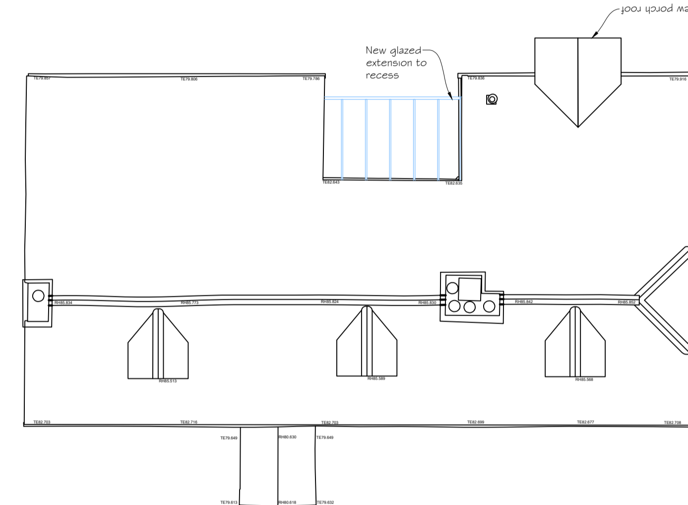
5 Roof Plan 1 : 100
