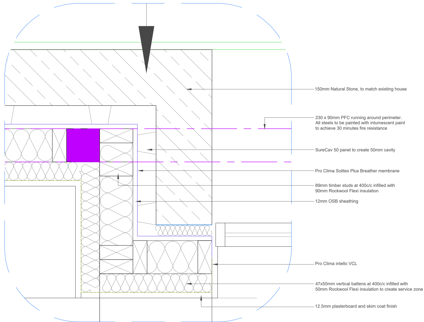
Detail 01 Jamb
