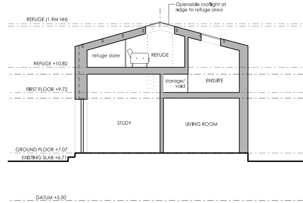
SECTION AA' 1:50 @A1
