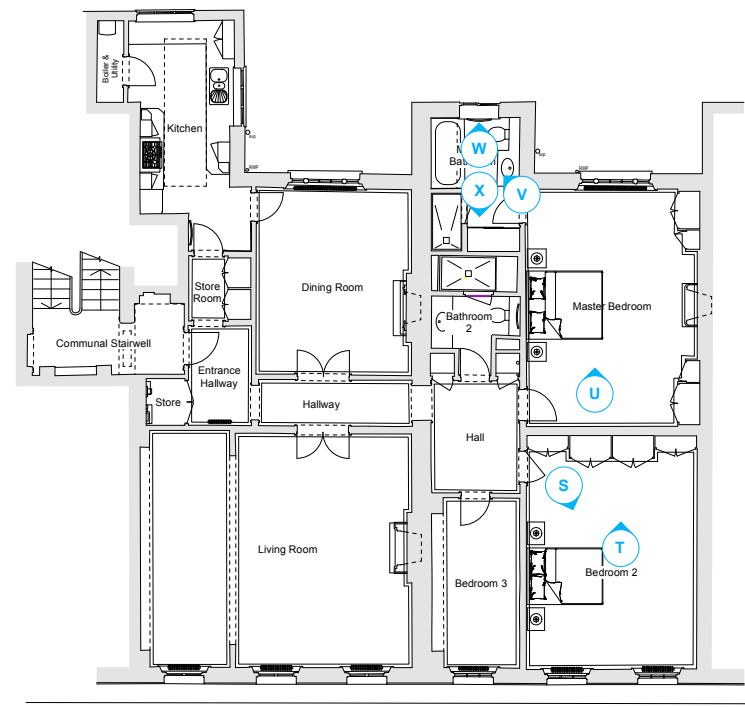
KEYPLAN 1 1:200 @ A3
