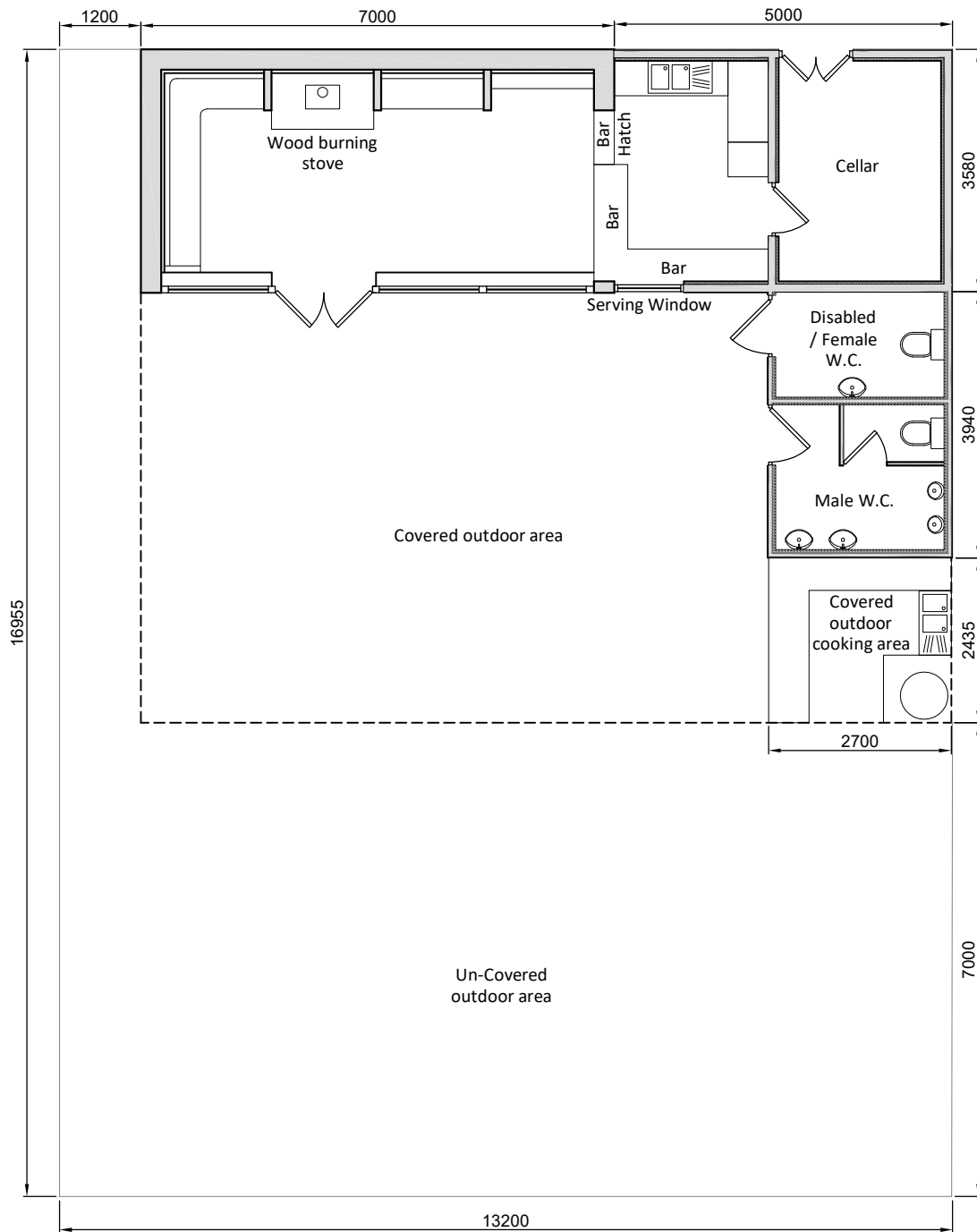
TAP BAR PLAN 1:100 @ A4
