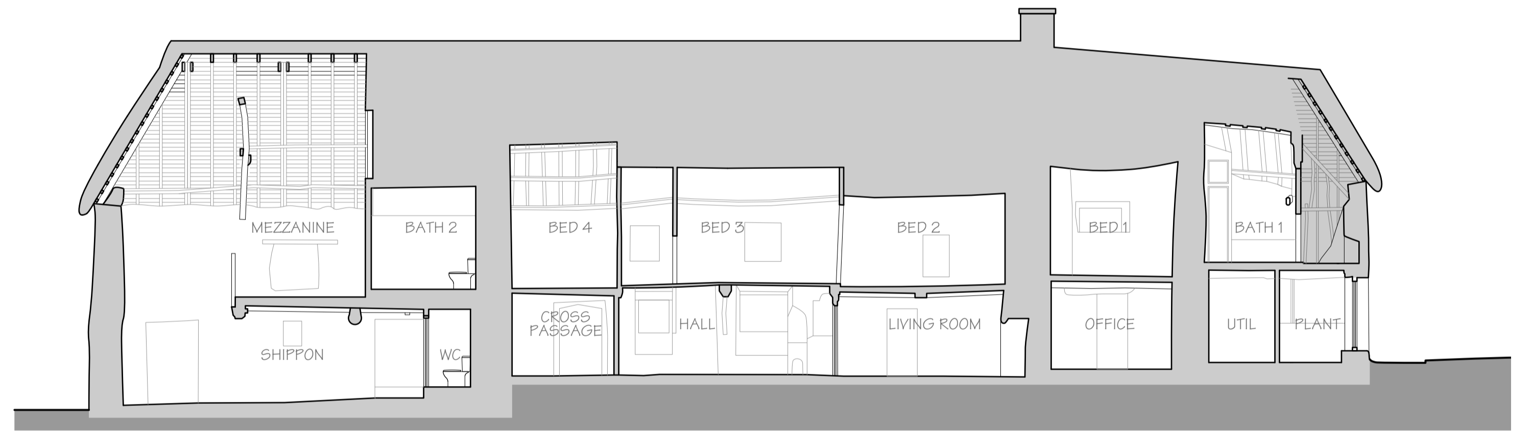
SECTION A-A
