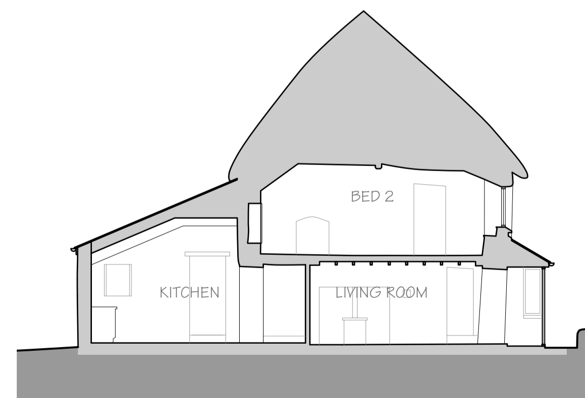
SECTION D-D
