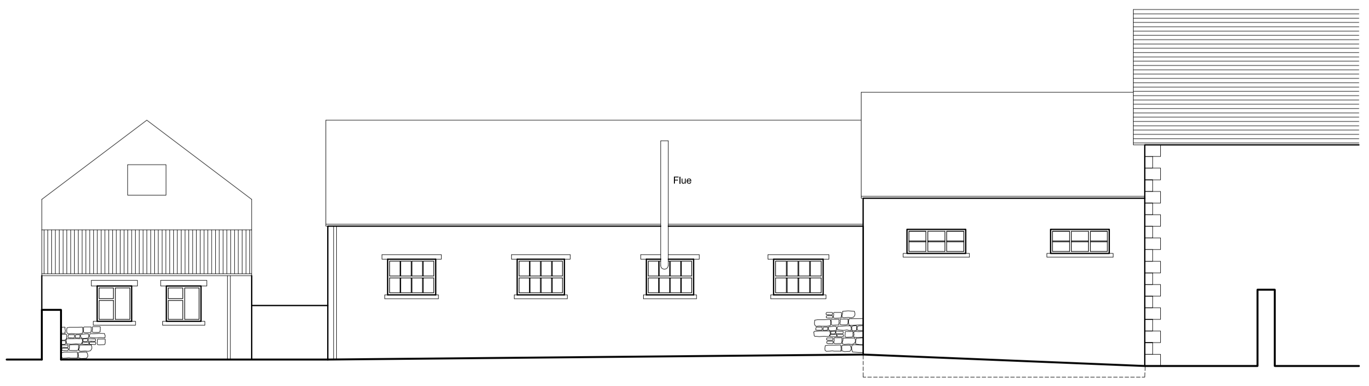
Elevation 7
