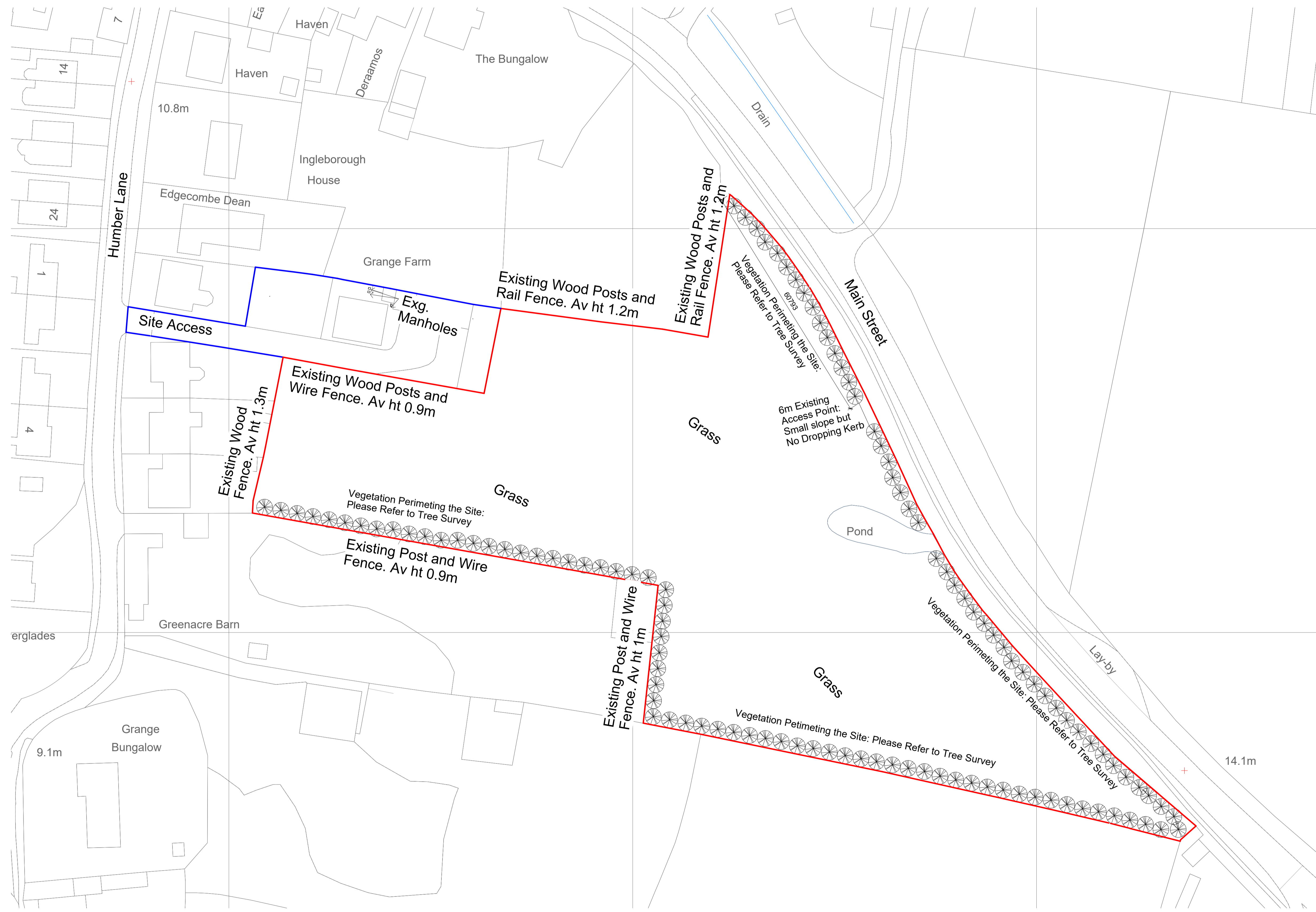
Existing Site Plan 1 : 500
