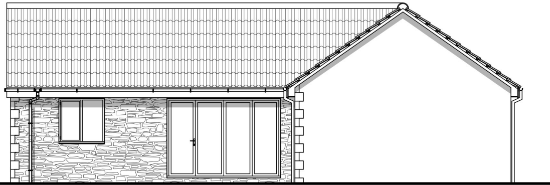
ELEVATION A
