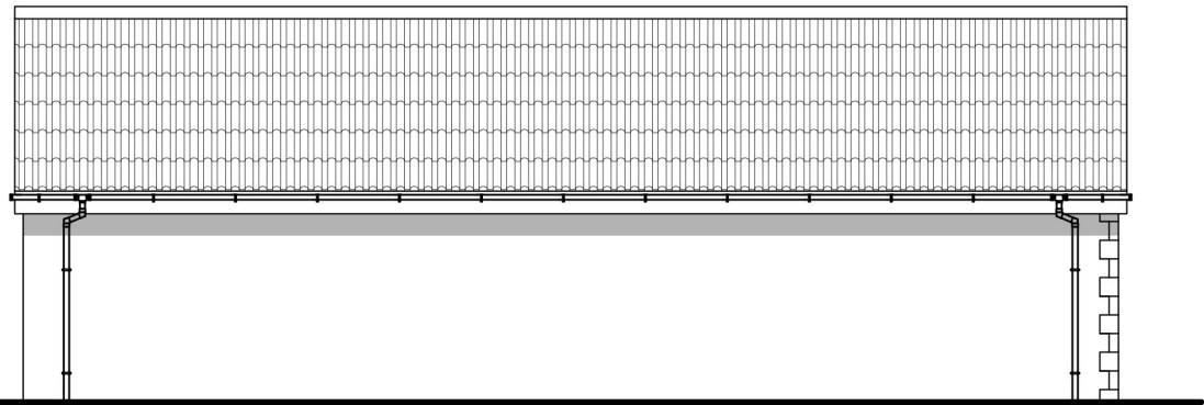
ELEVATION B
